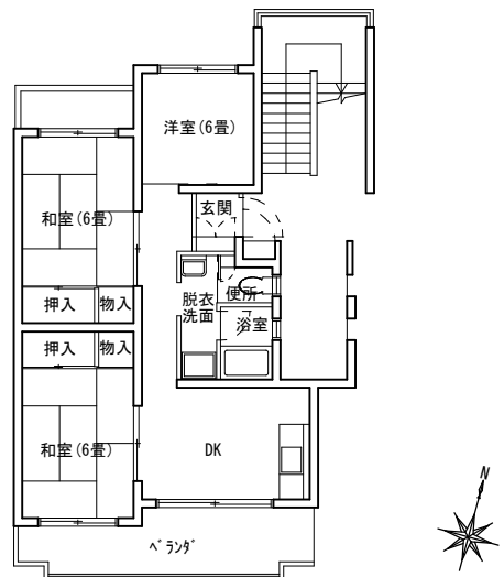
第2住宅 (3DK)
